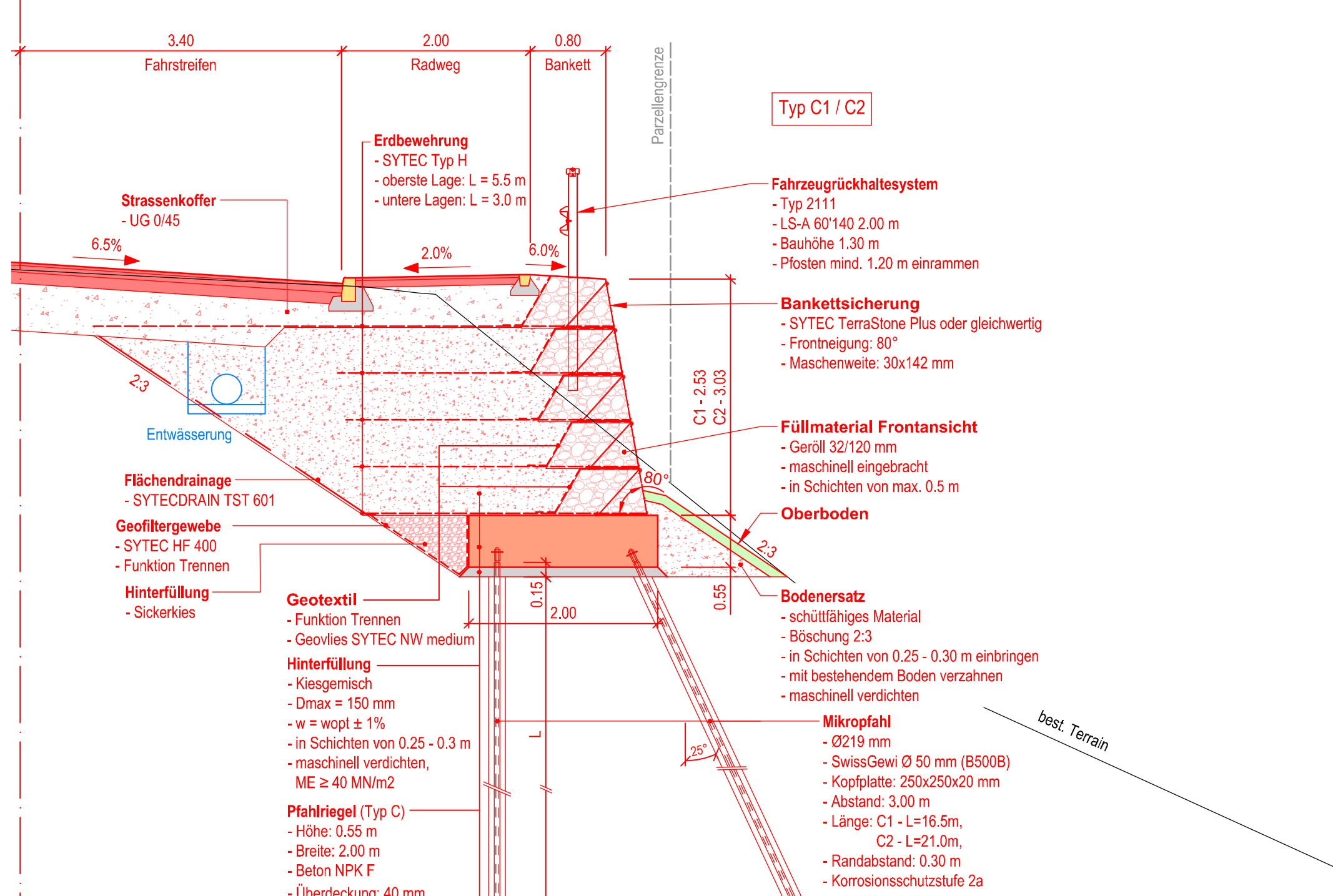
Schnitt C-C 1:50
