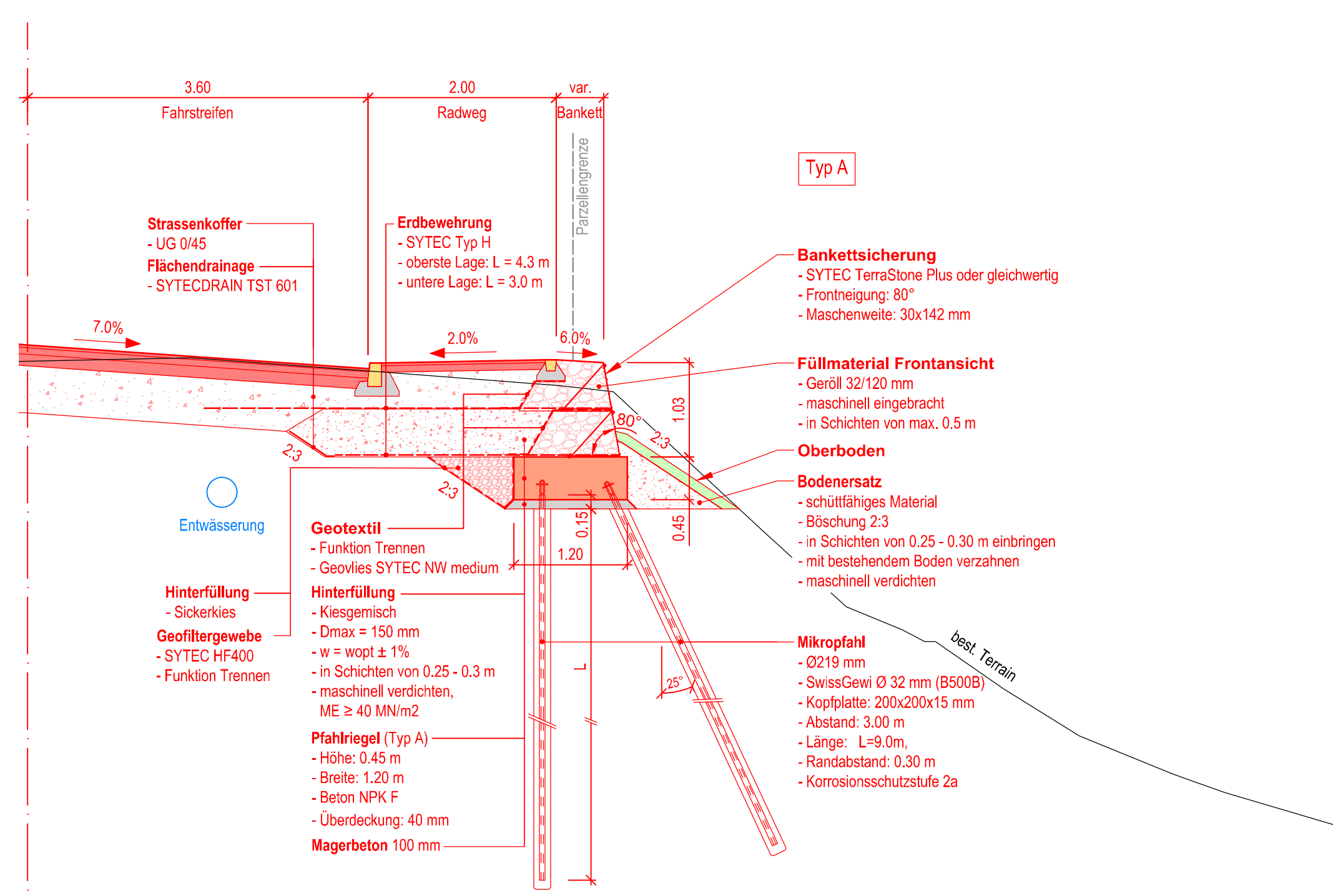
Schnitt A-A 1:50
