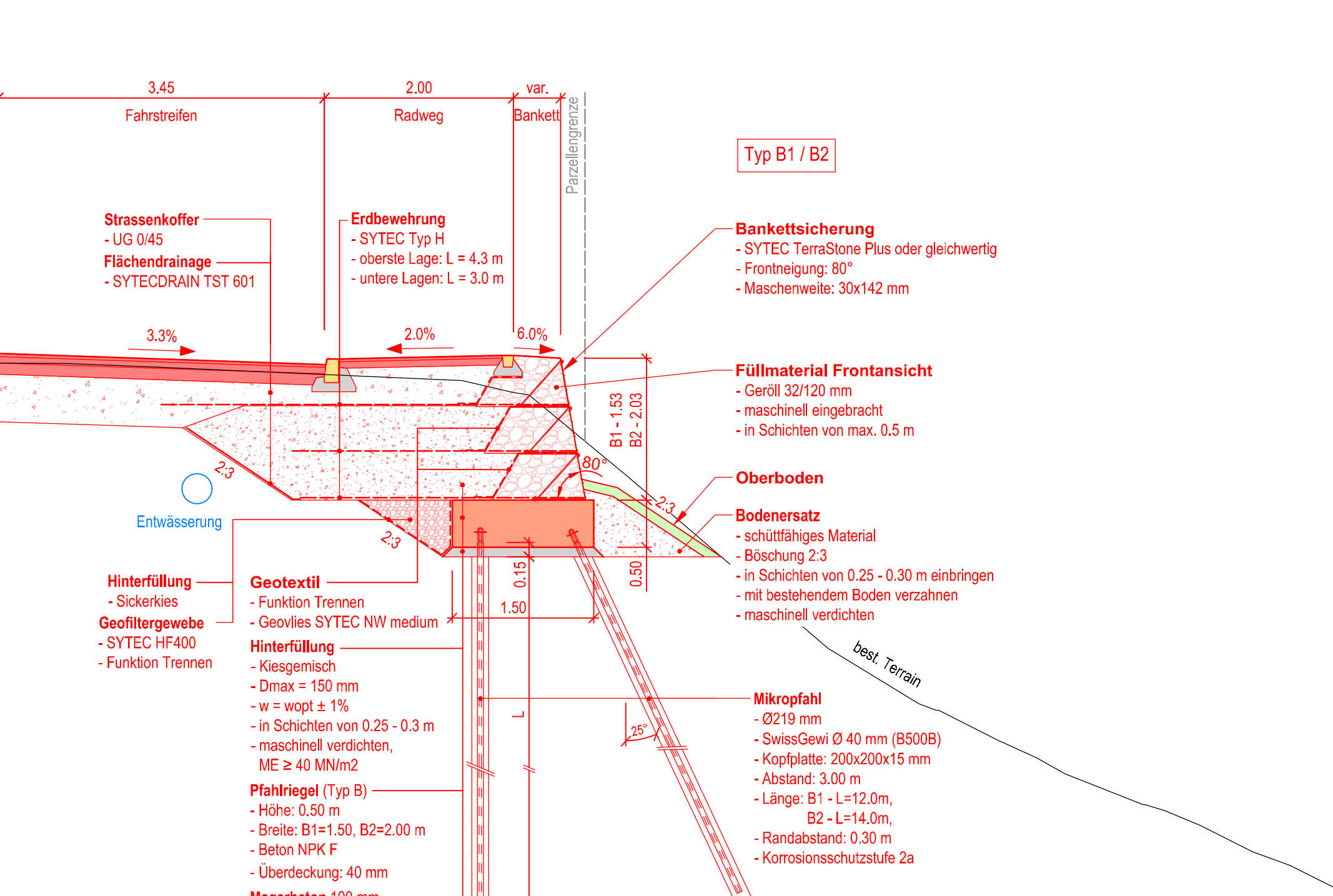
Schnitt B-B 1:50
